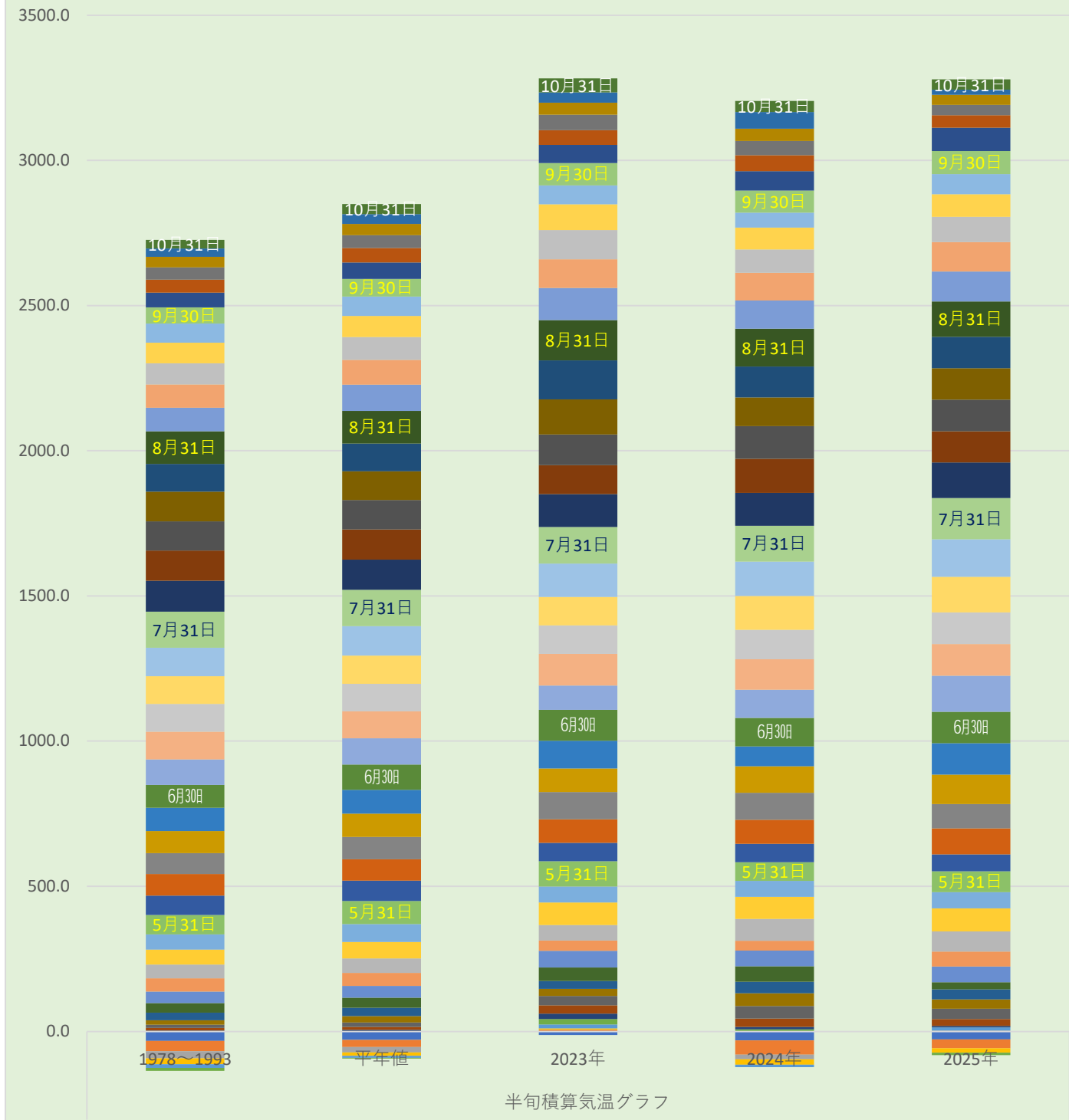
名寄市の3～10月 半旬積算気温（平均気温×日数）
