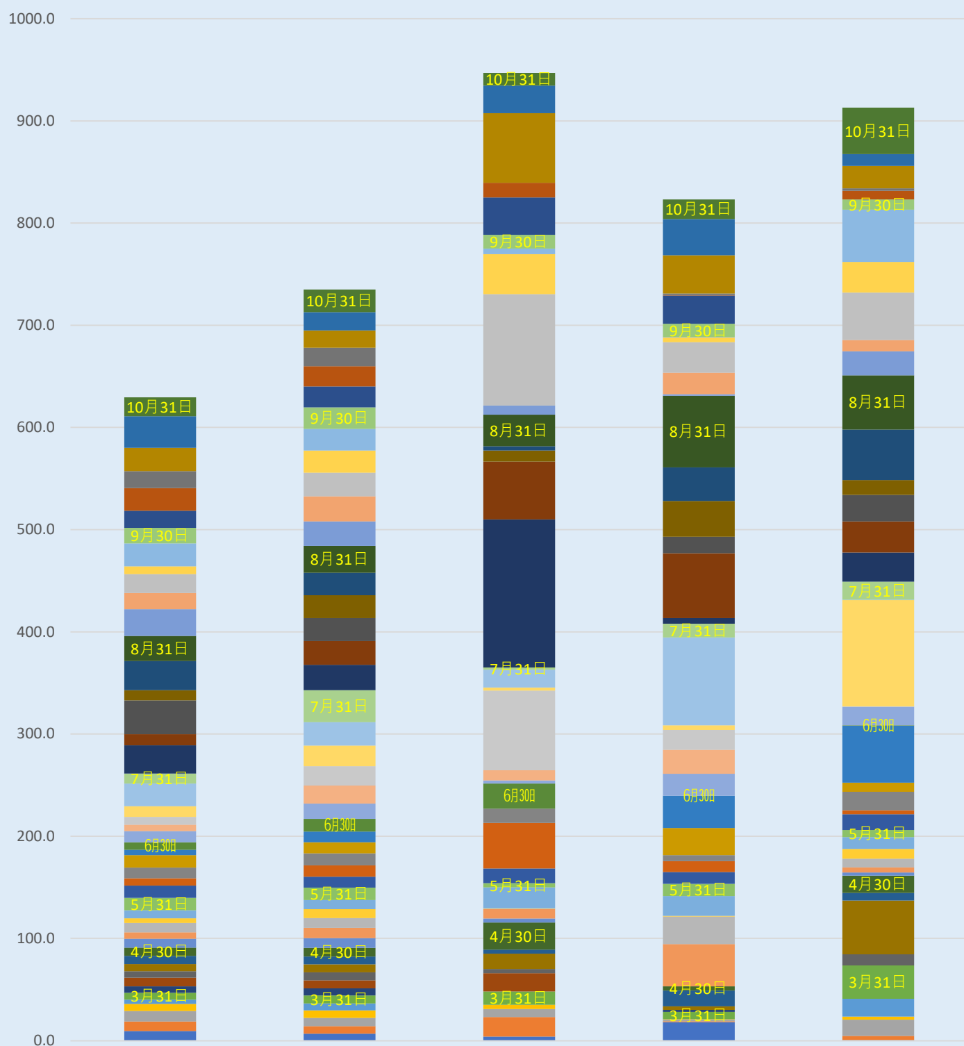
名寄市の3～10月 半旬降水量
